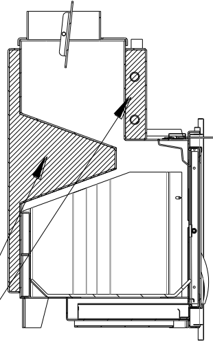
SECCIÓN A-A ESCALA 1 : 15
