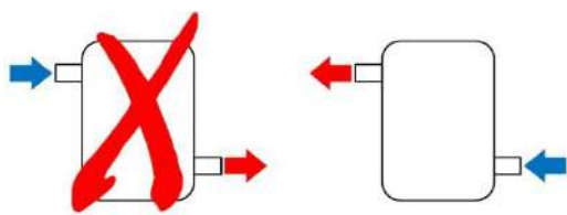
Figura nº10 - Ligação incorreta (esquerda) e ligação correta (direita)
