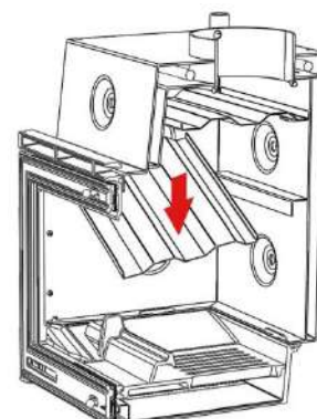
Figura nº17 - Desmontagem do defletor inferior Sarria Sakan 20
