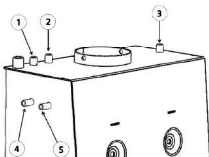
Figura nº13 - Uniões de ligação na serpentina permutadora de calor
