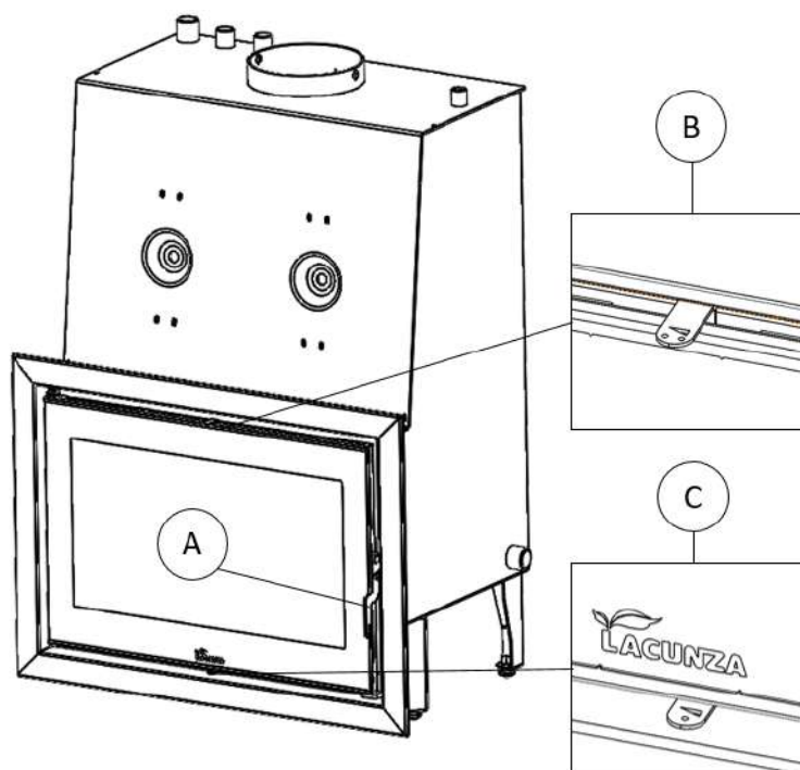
Figura nº15 - Elementos de funcionamento do aparelho
