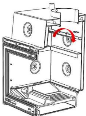
Figura nº18 - Desmontagem do defletor superior Sarria Sakan 20
