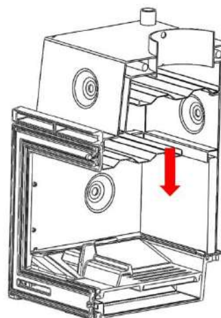
Figura nº5 - Meter a peça girando e empurrando para cima até soltar a pestana inferior e deixar cair
