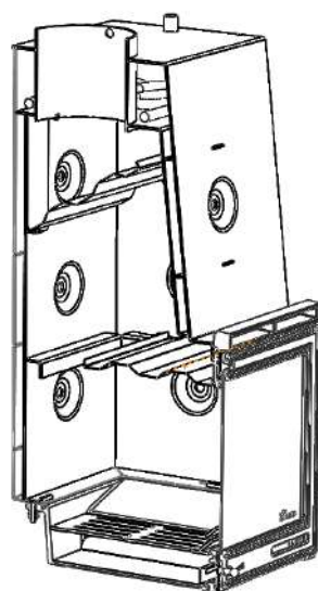
Figura nº19 - Vista de secção com dois defletores instalados (Sarria Sakan 20)
