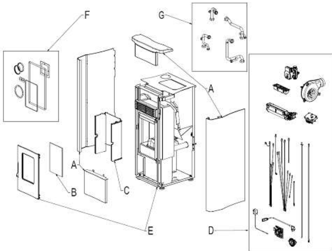
Fig. 1 - Desenho explodido
