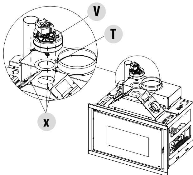
Figura 7– Posizione morsetti ventilatori
