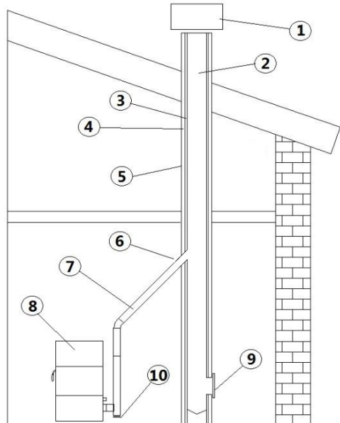
Fig. 5 - Componentes da chaminé
