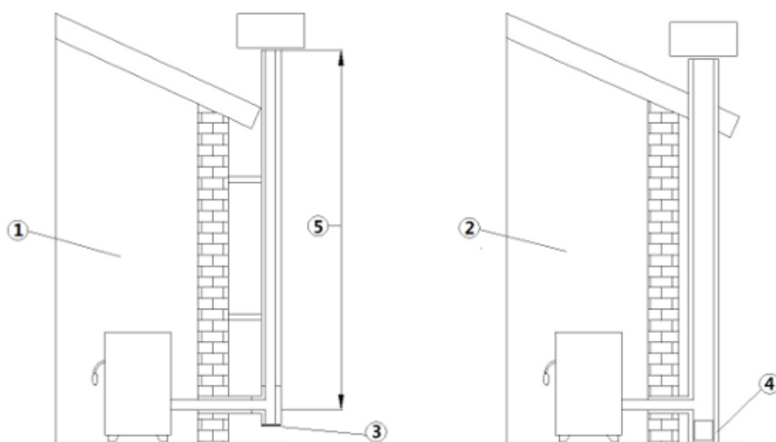
Fig. 1 - Conduas de evacuação de fumos
