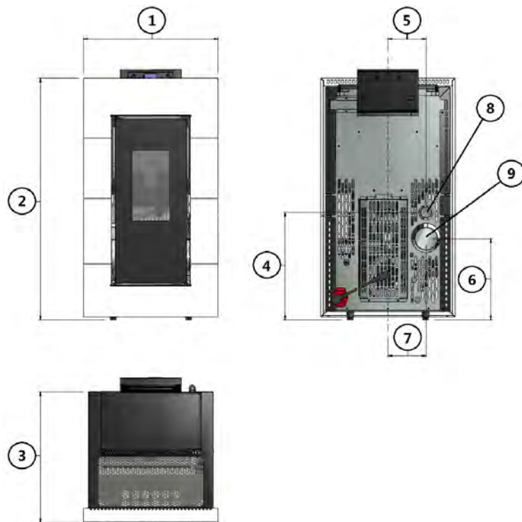
Fig. 14 - Dimensões gerais: Kami
