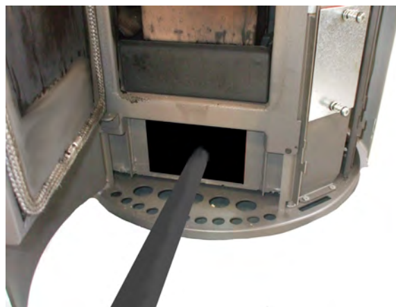
Fig. 36 - Limpeza da câmara de fumos
