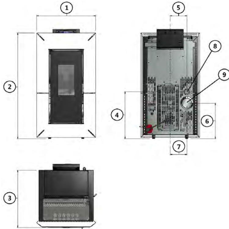
Fig. 13 - Dimensões gerais: Mika
