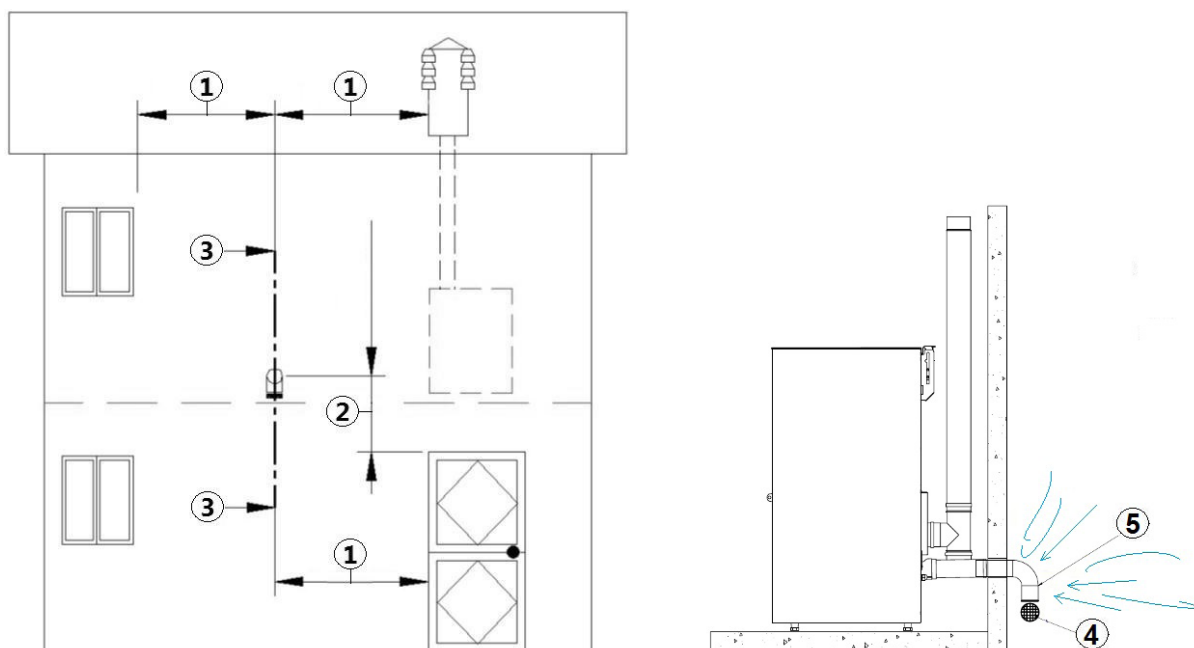
Fig. 7 - Tomada de ar para a instalação
